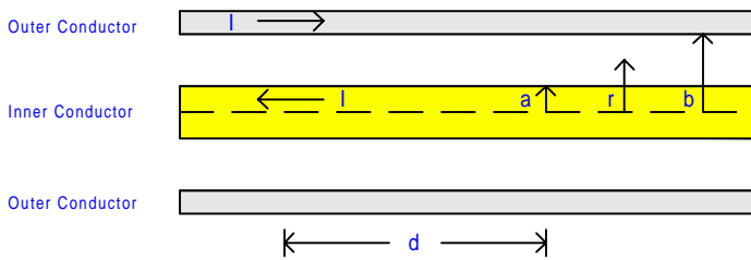
Longitudinal Section
